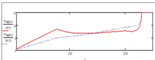
16. ábra. A bontófog hosszanti keresztmetszetének analitikus modellezéssel kapott optimális alakja
