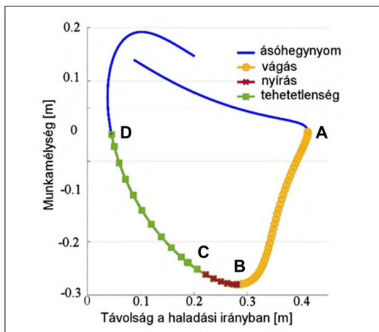
2. ábra. Egy ásóél csúcspontjának pályája
