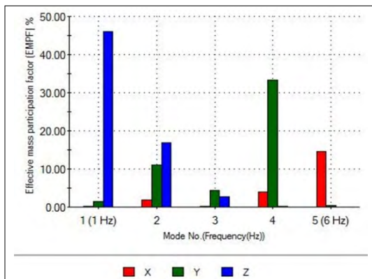
14. ábra. Frekvenciaválasz-diagram
