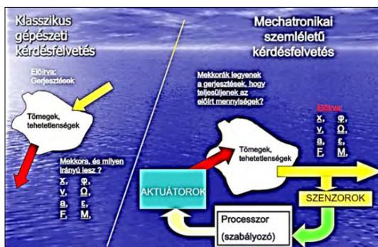
2. ábra. Hagományos/mechatronikai szemléletű tervezés összehasonlítása
