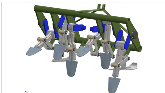
1. ábra. MSS-1,40M-ásógép szerelési modellje
