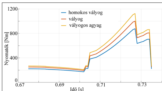
5. ábra. Egy ásó nyomatékszükséglete egy fordulat alatt
