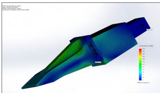
17. ábra. Bontófog végeelem-módszerrel való optimalizálása
