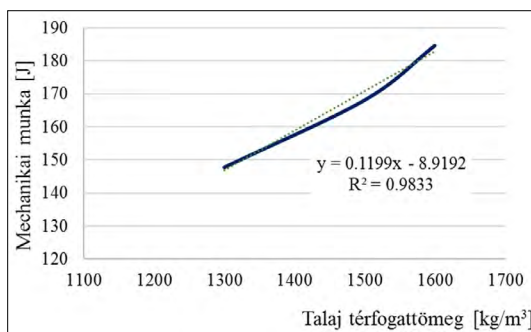
6. ábra. Ásásmechanikai munka igénye és a talaj térfogattömegének összefüggése
