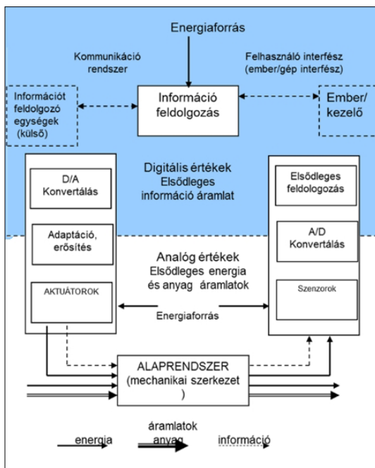
3. ábra. A mechatronikai szemléletű tervezésben alkalmazott áramlatok
