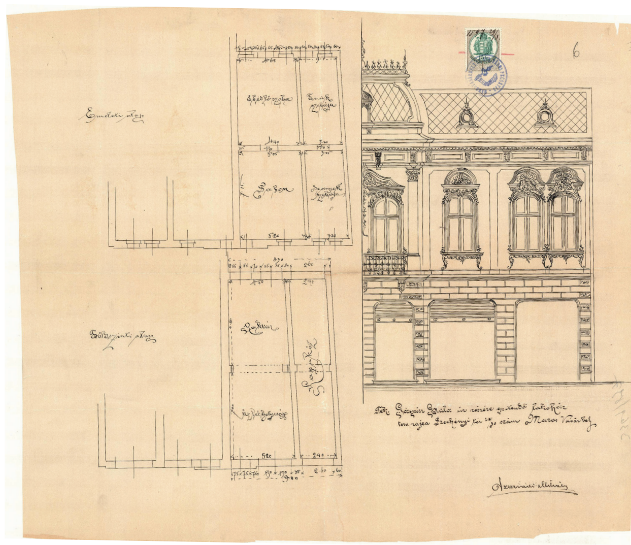
7. Átalakítási terv Gáspár Gyula házához, 1897 / Conversion plan of the house of Gyula Gáspár, 1897 (SJAN Mureş, Consiliul oraşului, 3369/1897)
