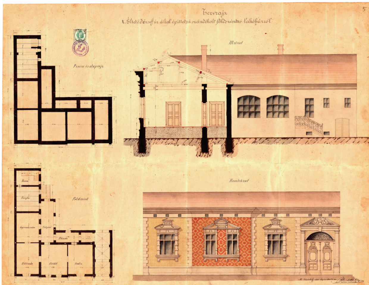
20. Élteső József házának tervrajza, 1896 / Plan of the house of József Élteső, 1896 (SJAN Mureș, Consiliul orașului, 6617/1897)
