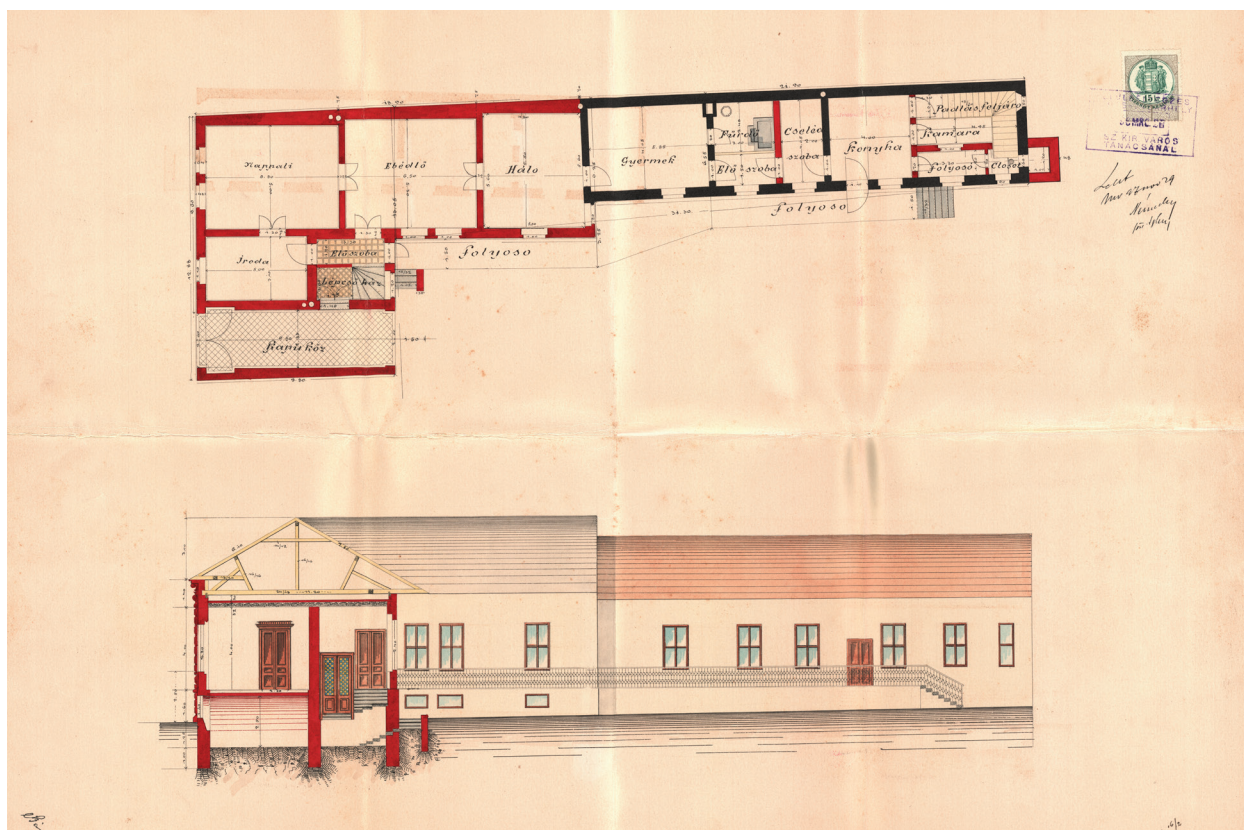
16. Bányai Béla házának alaprajza és hosszmetszete, 1896 / Ground plan and longitudinal section of the house of Béla Bányai, 1896 (SJAN Mureş, Consiliul oraşului, 3052/1896)
