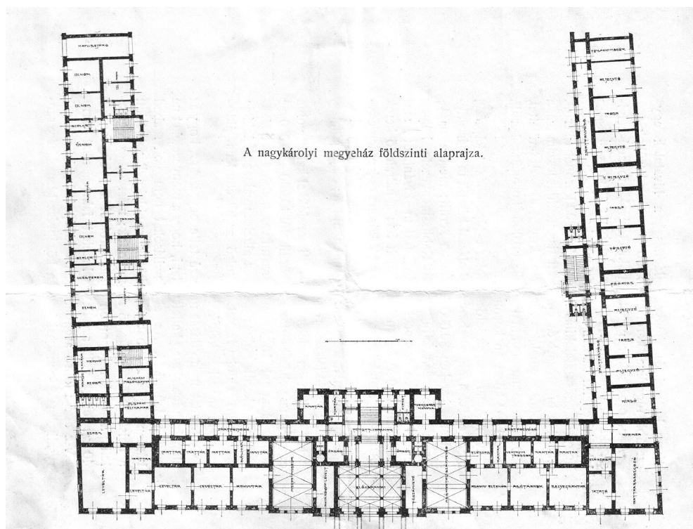
12. kép. A megyeház földszinti alaprajza, Schodits Lajos, 1904 ( Építő Ipar 31. 30. [1907. július 28.] 293)
