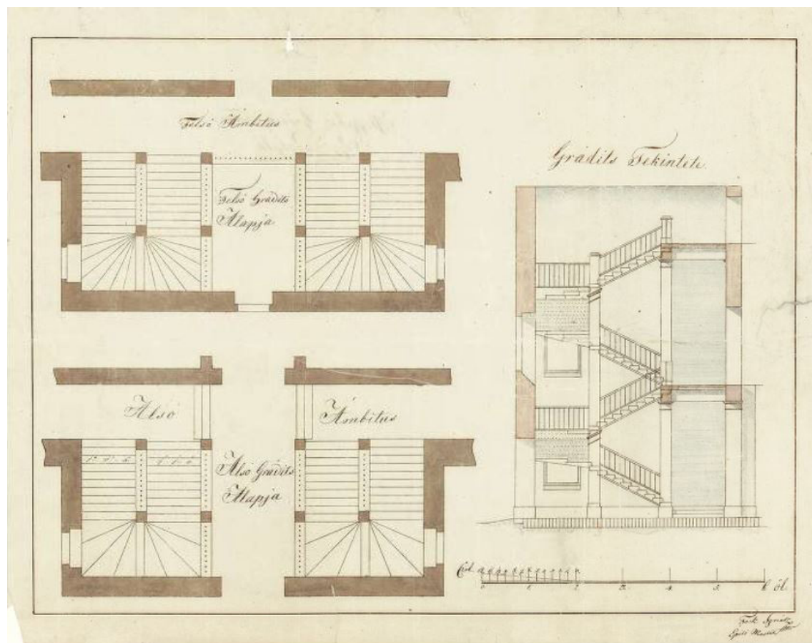
5. kép. A vármegye-ház lépcsőházának tervrajza, Fock Ignác, 1854 (BFL-YBL TERV, No. 19/10) Fig. 5. Plan of the stairway in the county hall, Ignác Fock, 1854 (BFL-YBL TERV, No. 19/10)
