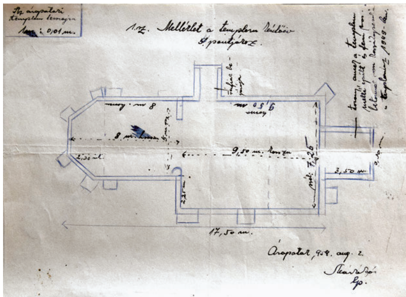
1. Árpátság, a református templom alaprajza
