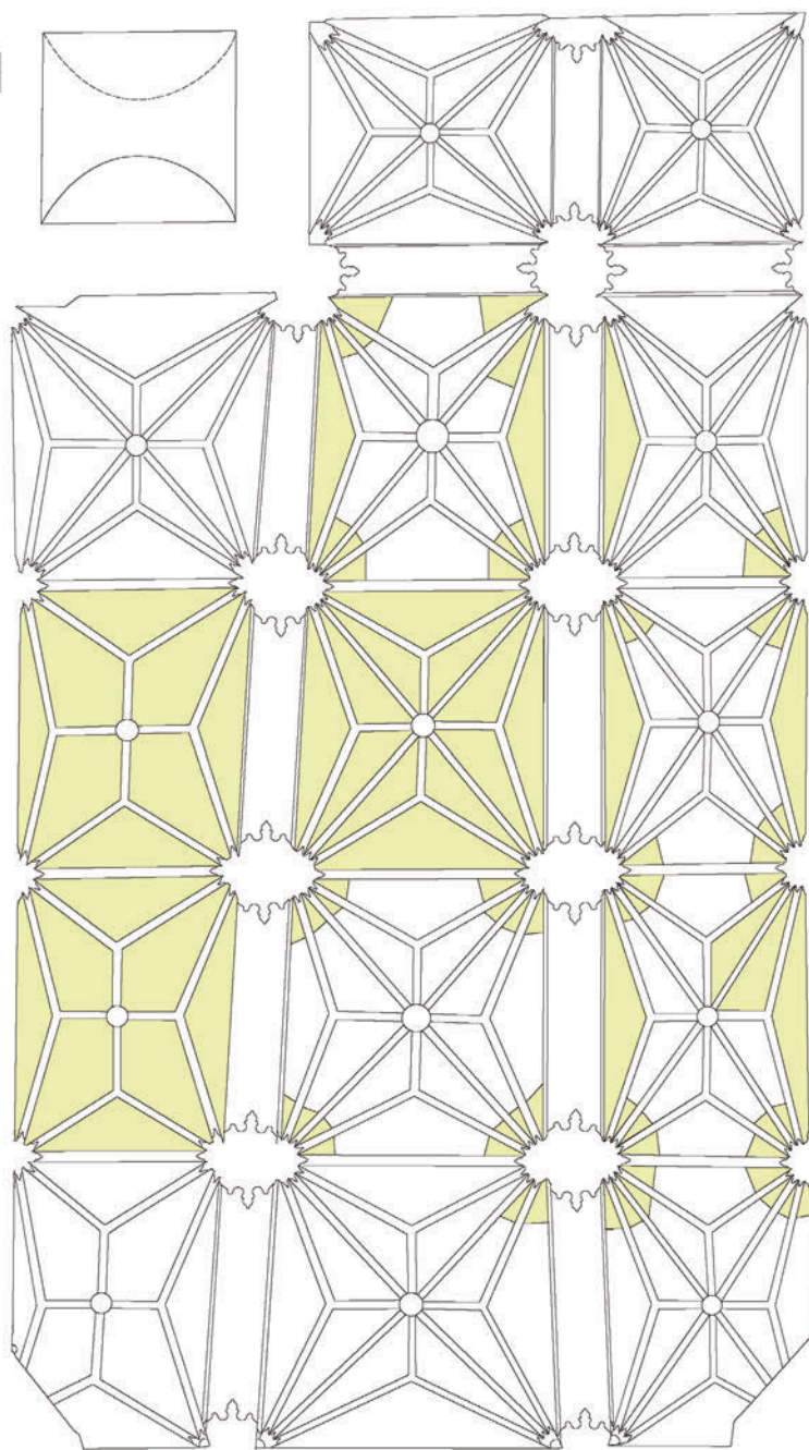
10. A hosszház boltmezőinek falazása, sárgával a kővel falazott süvegek, sötétszürkével a vaspántok. A szerző vázlata, 2020
