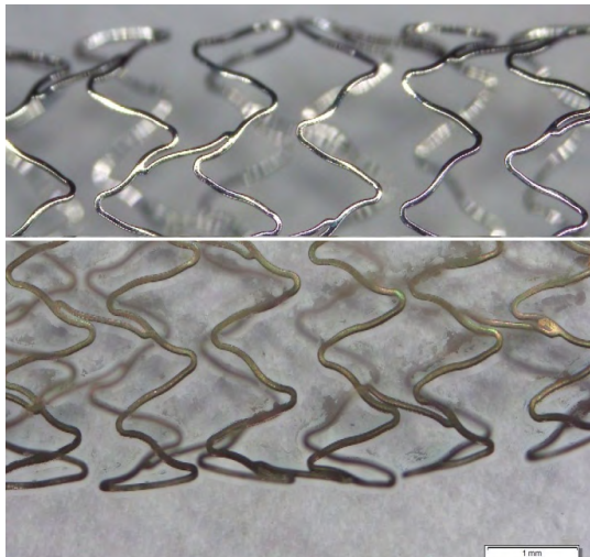
3. ábra. A sztent felülete a korróziós kísérlet előtt (feletül) és után (alul)
